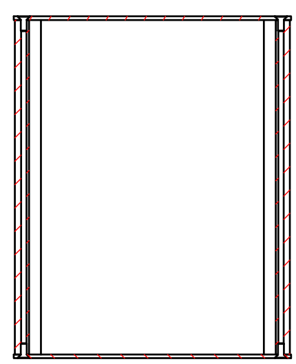
C-C ( 1 : 3.5 )
