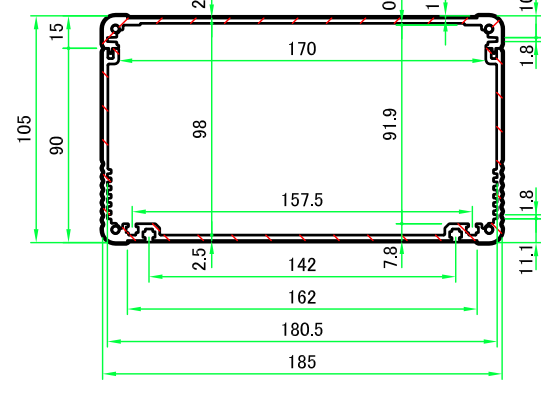
A-A ( 1 : 3.5 )
